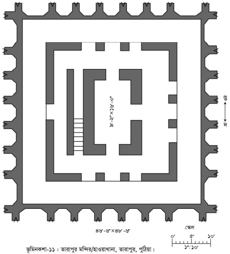
ভূমিকশা-১১ : ভাৰাপুৰ মন্দিৰ/হাওয়ামান, ভাৰাপুৰ, পুঠিয়া।
